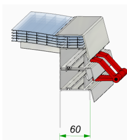
Profilo freddo standard
