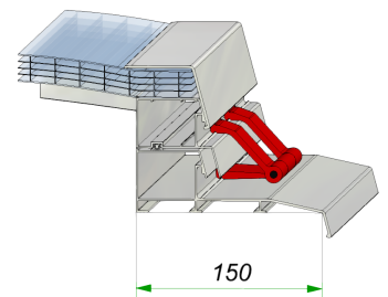
Profilo freddo per cordolo largo
