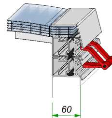
Profilo taglio termico (TT)
